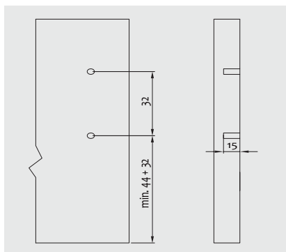
Димензии за бушење на лицето
