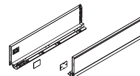
Метални страници Slim Box 1900 (пар) со висина 118 мм
