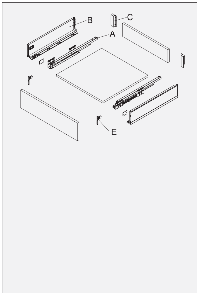
Пар лизгачи за Slim Box 1900
