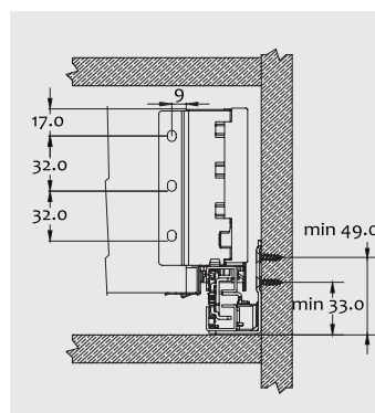
Димензии за монтажа на задниот панел
