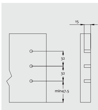
Димензии за бушење на лицето
