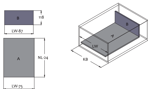
Димензии за сечење на панелите
