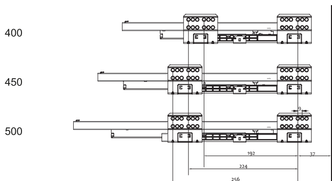
Димензии за монтажа на лизгачите
