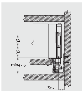
Димензии за монтажа на држачот за лице
