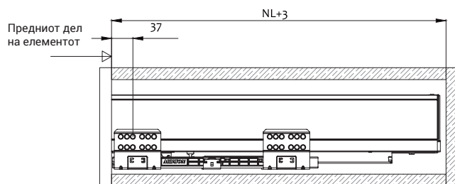
Просторни барања на фиоката
