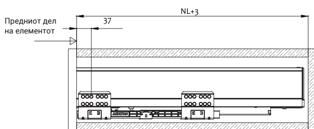
Просторни барања на фиоката
