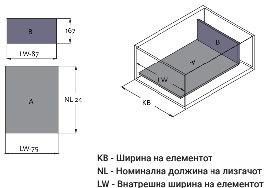
Димензии за сечење на панелите
