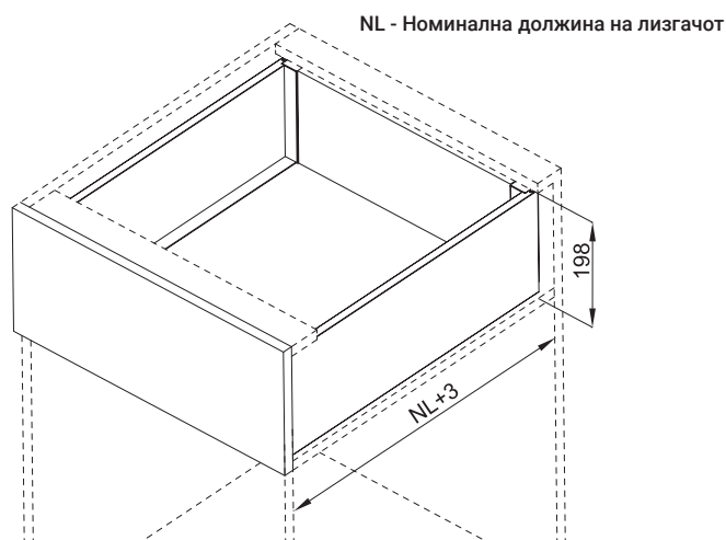
Просторни барања на фиоката
