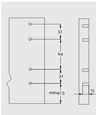
Димензии за бушење на лицето
