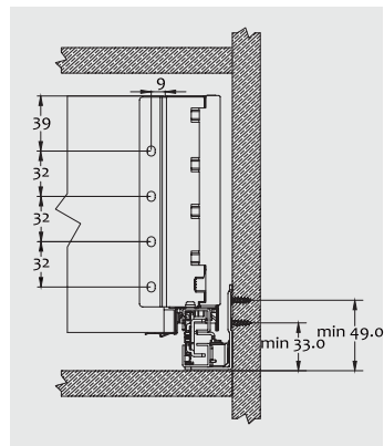
Димензии за монтажа на задниот панел
