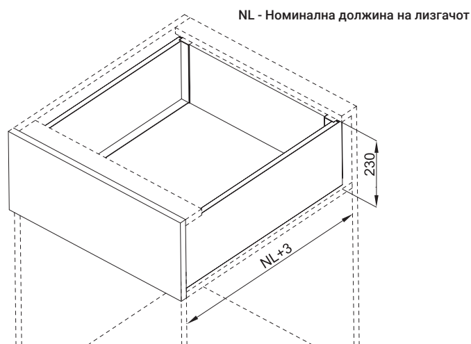
Просторни барања на фиоката
