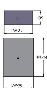
Димензии за сечење на панелите
