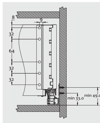
Димензии за монтажа на задниот панел
