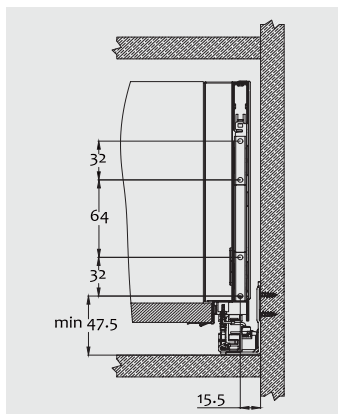
Димензии за монтажа на држачот за лице
